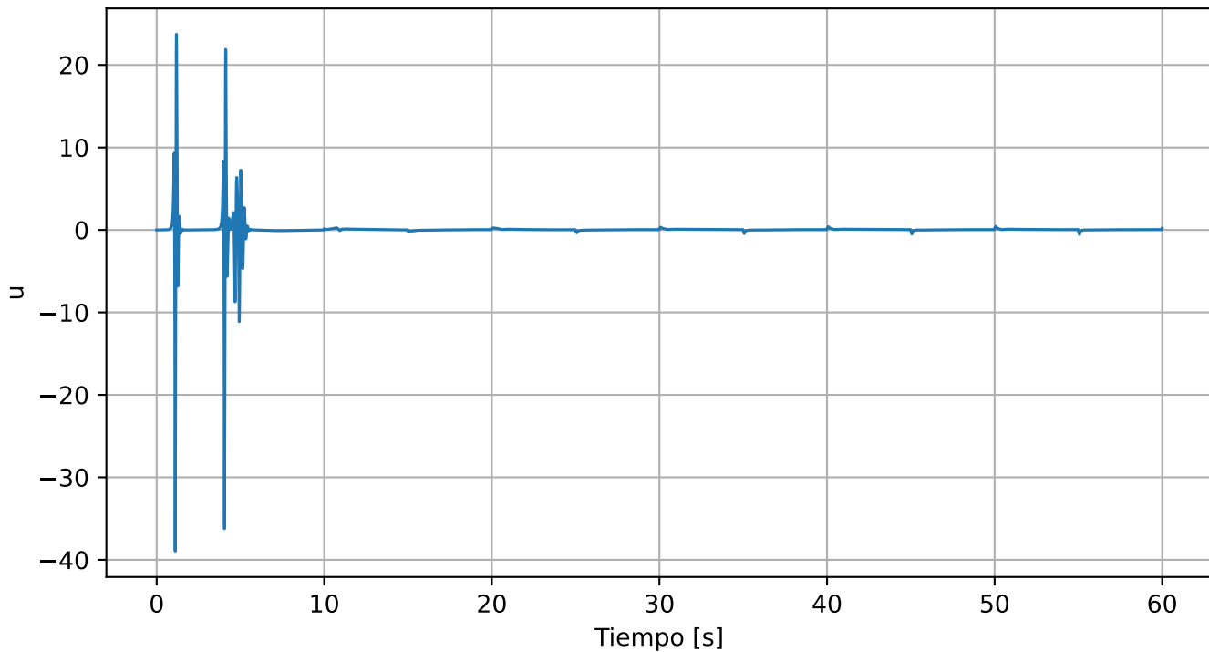
Señal de control MRAC - tren de pulsos
